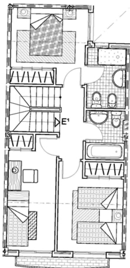
PLANTA PISO 1º
