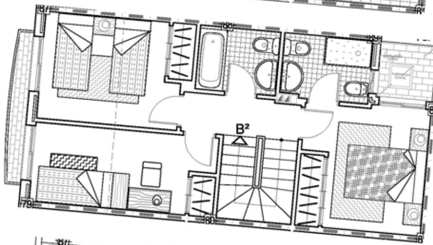
PLANTA PISO 1º
