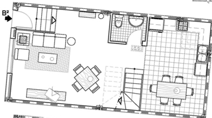
PLANTA BAJA
